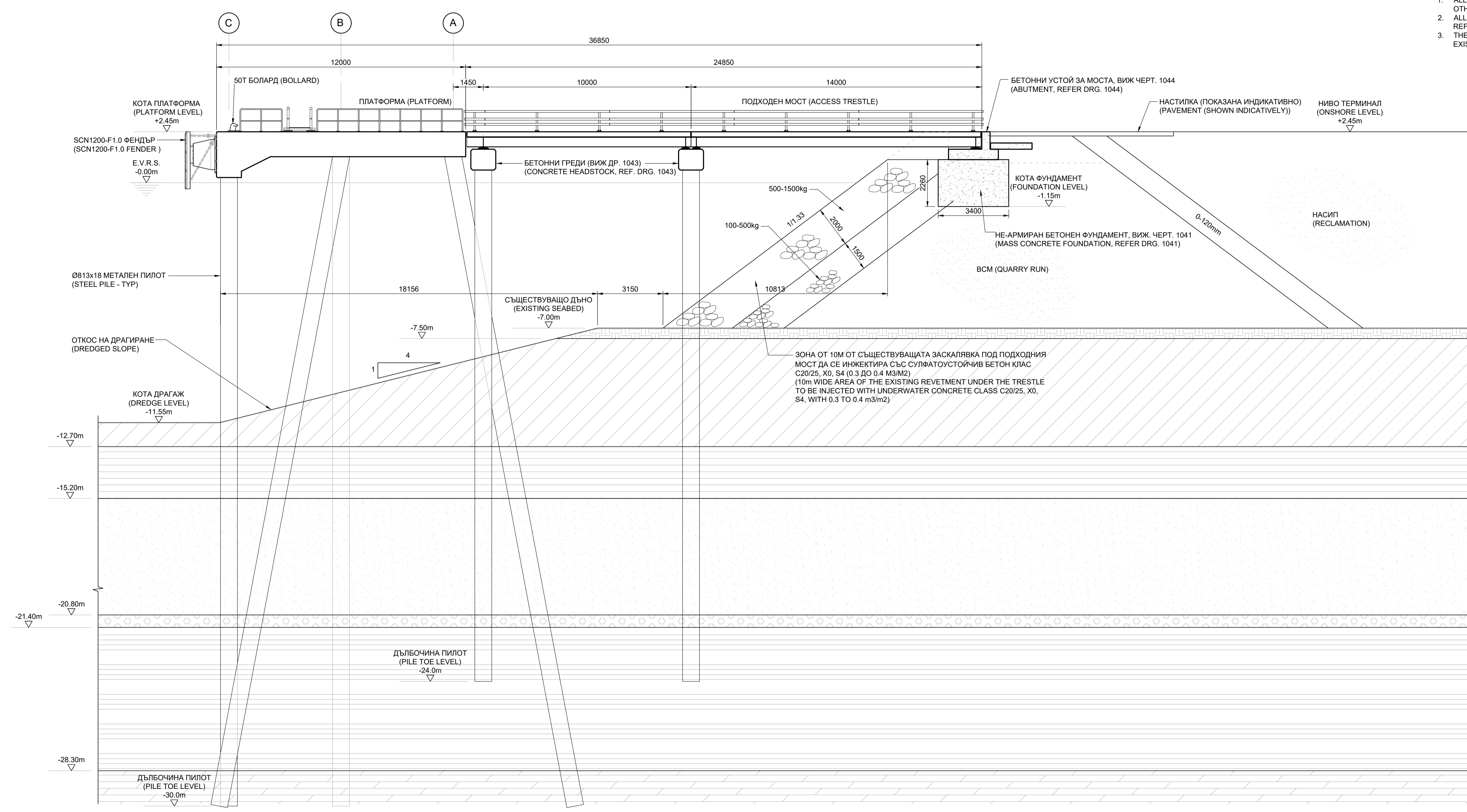
ПЛАТФОРМА - ТИПОВ РАЗРЕЗ (PLATFORM - TYPICAL SECTION) 1:100
